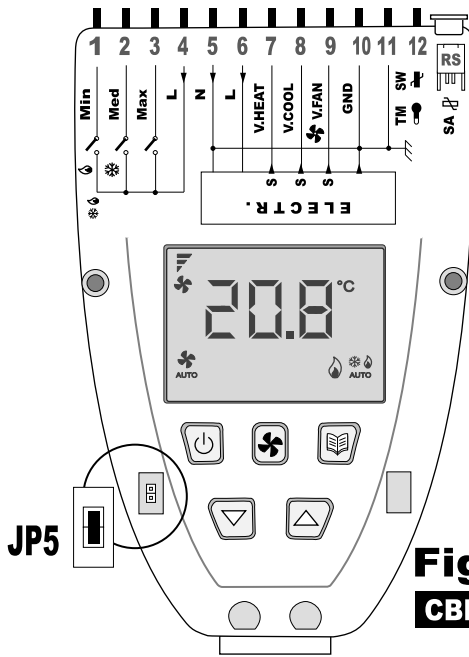
Schema elettrico interno Internal wiring diagram
