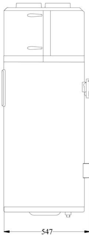
VISTA LATERALE (mm)
