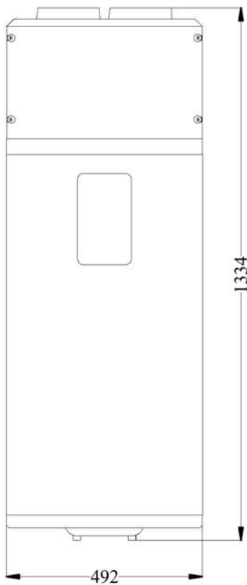
VISTA FRONTALE (mm)
