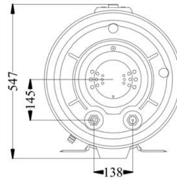
VISTA INFERIORE (mm)
