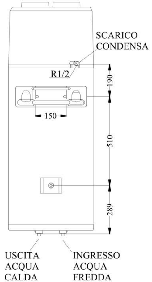
VISTA POSTERIORE (mm)
